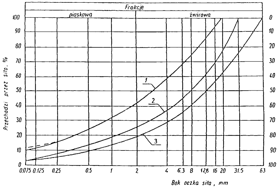
Rysunek 1. Pole dobrego uziarnienia kruszyw przeznaczonych na podbudowę wykonywane metodą stabilizacji mechanicznej 1-2 kruszywo na podbudowę zasadniczą (górną warstwę) lub podbudowę jednowarstw
