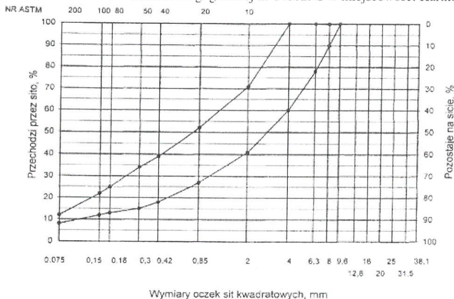
Rys. 3. Krzywe graniczne
