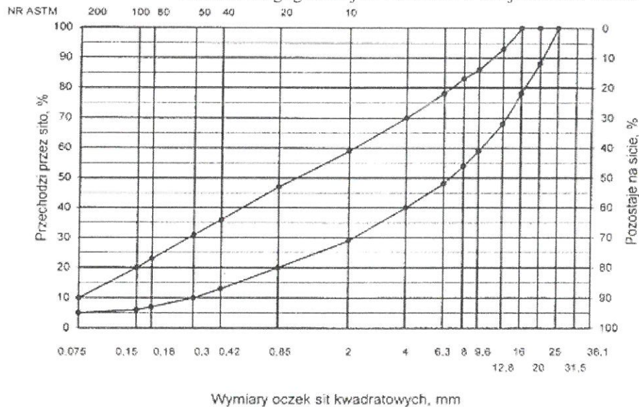
Rys. 1. Krzywe graniczne
