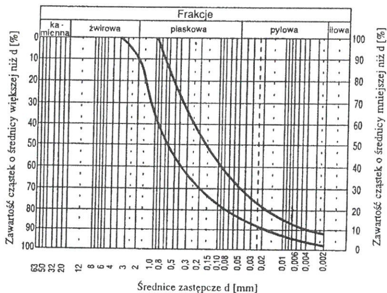
Rys. 1. Obszar mieszanki
