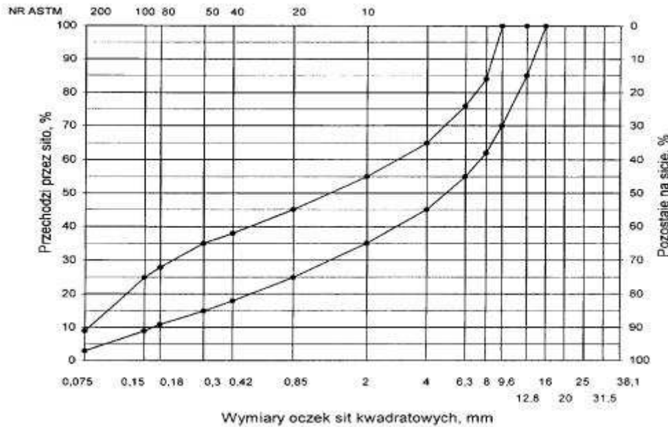
Rys. 10. Krzywe graniczne
