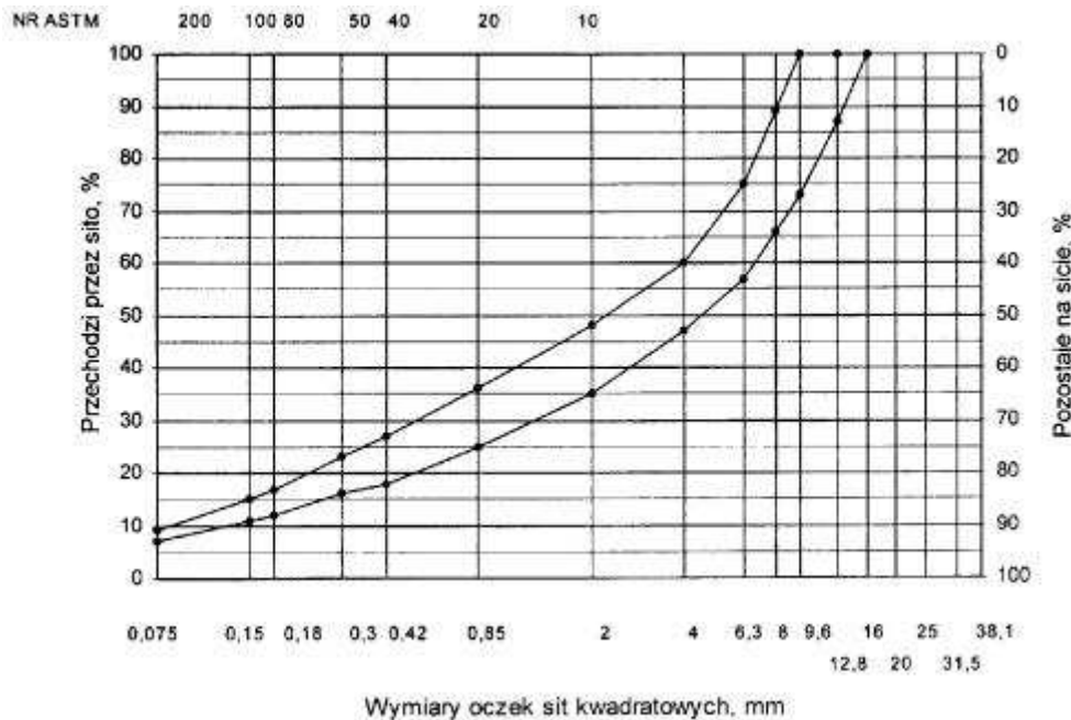
Rys. 7. Krzywe graniczne
