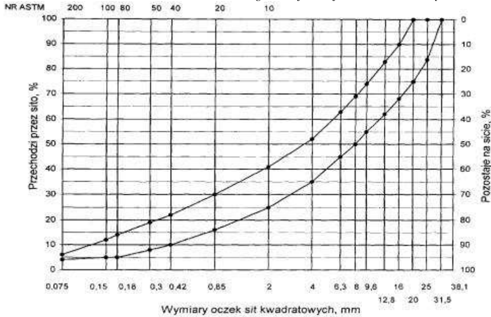
Rys. 11. Krzywe graniczne
