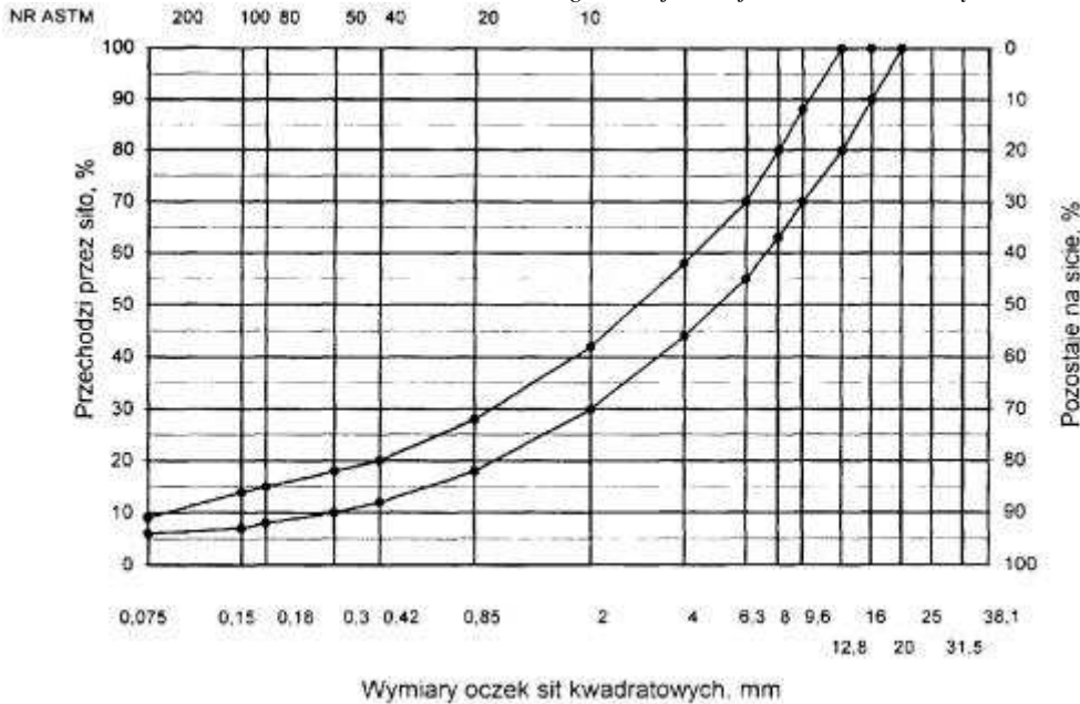
Rys. 6. Krzywe graniczne
