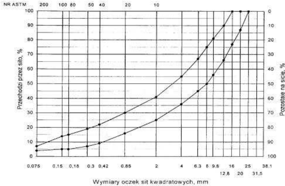
Rys. 12. Krzywe graniczne
