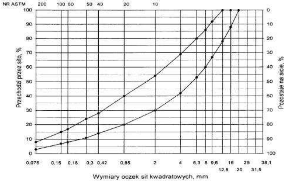
Rys. 9. Krzywe graniczne
